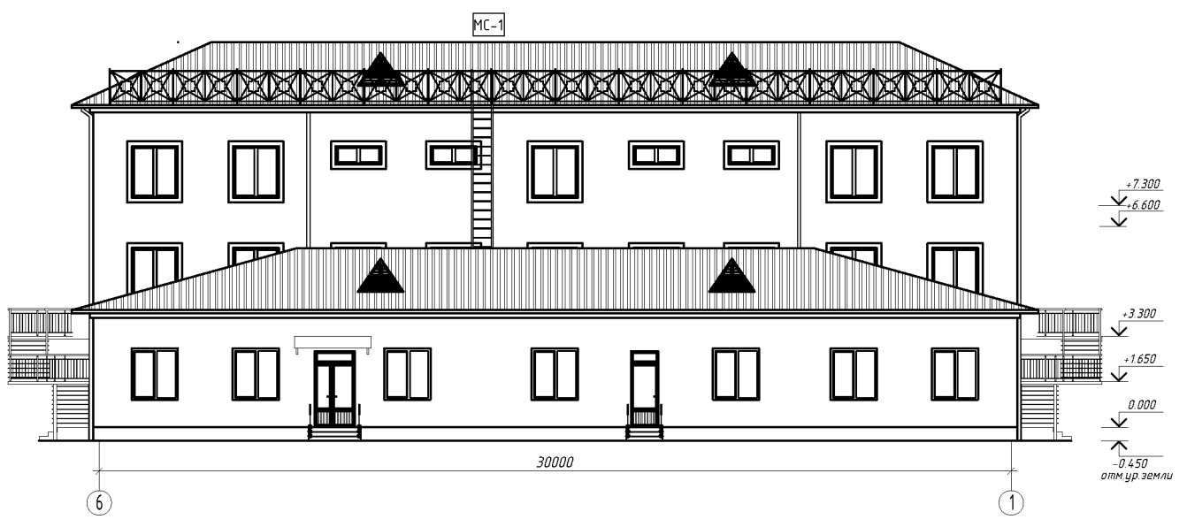
Фасад в осях 1-6
