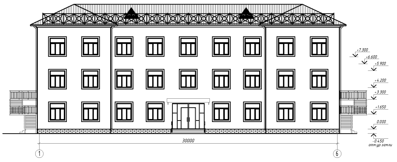
Фасад в осях 1-6
