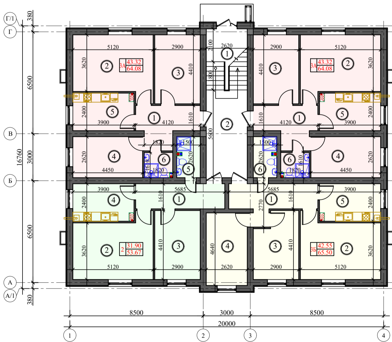
План 1-этажа
