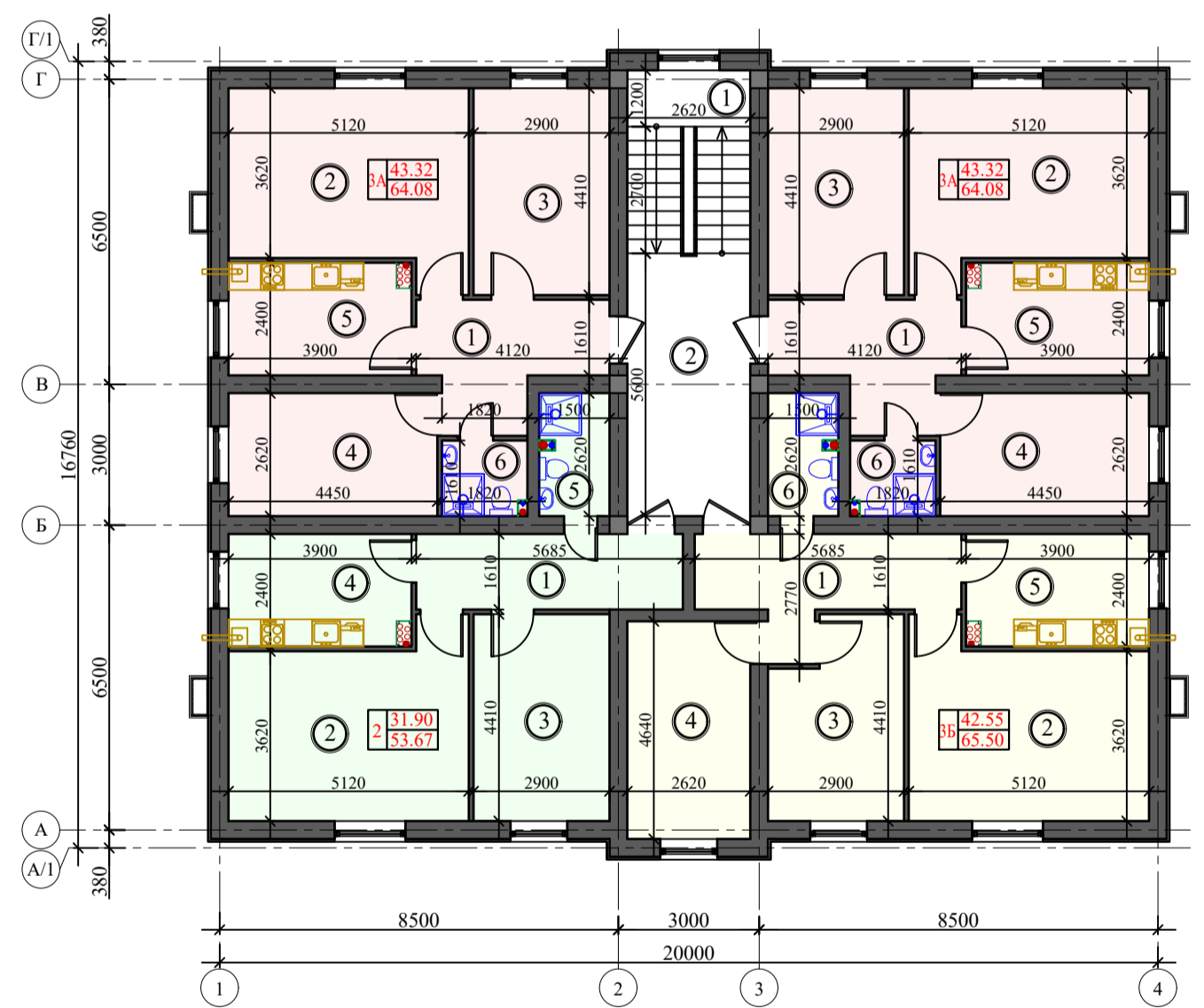
План 2-этажа
