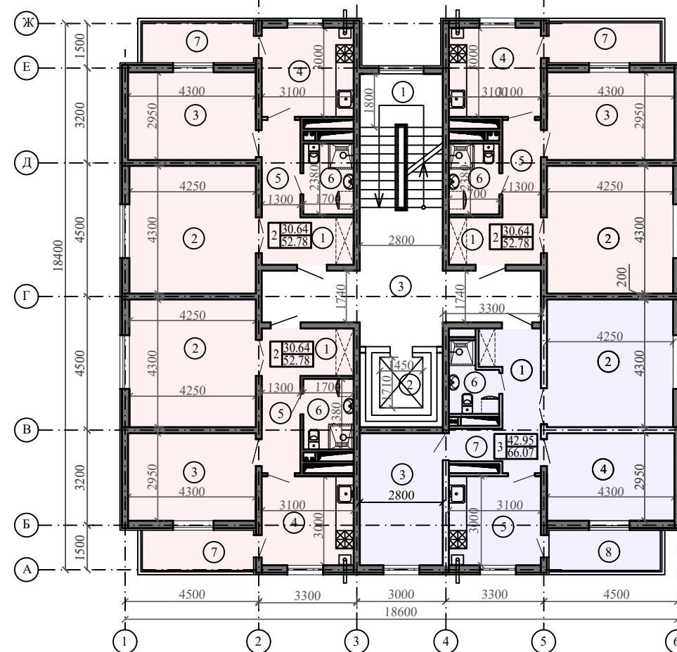
Намунавий қават тархи
