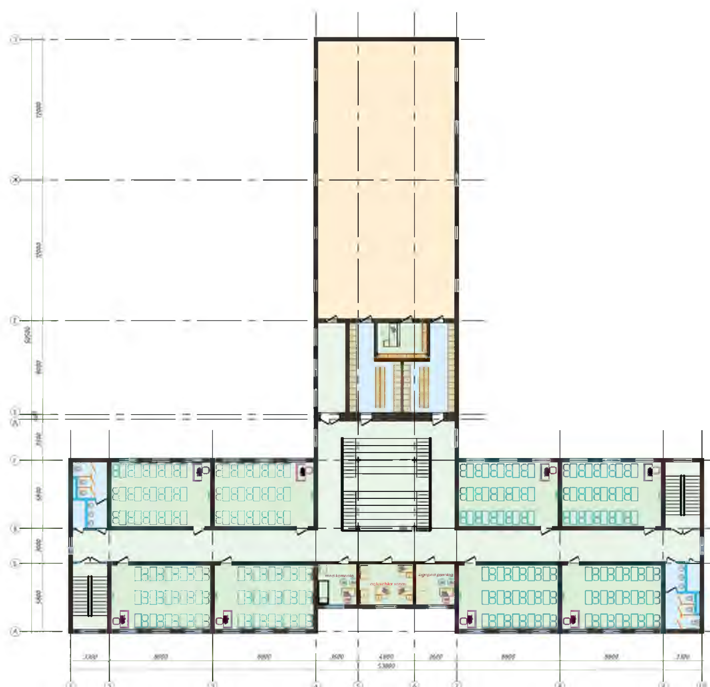
2-Қават тархи
