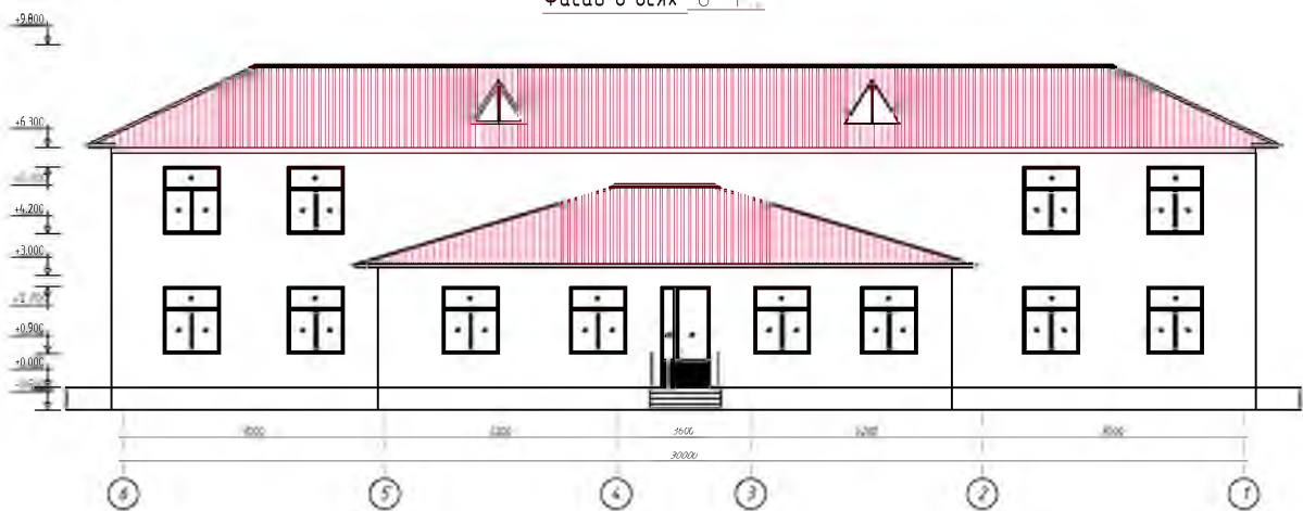
Фасад в осях "6-1".
