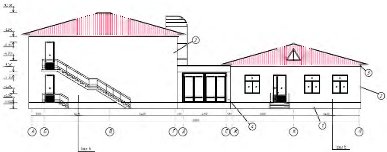
Фасад в осях "А-Л".
