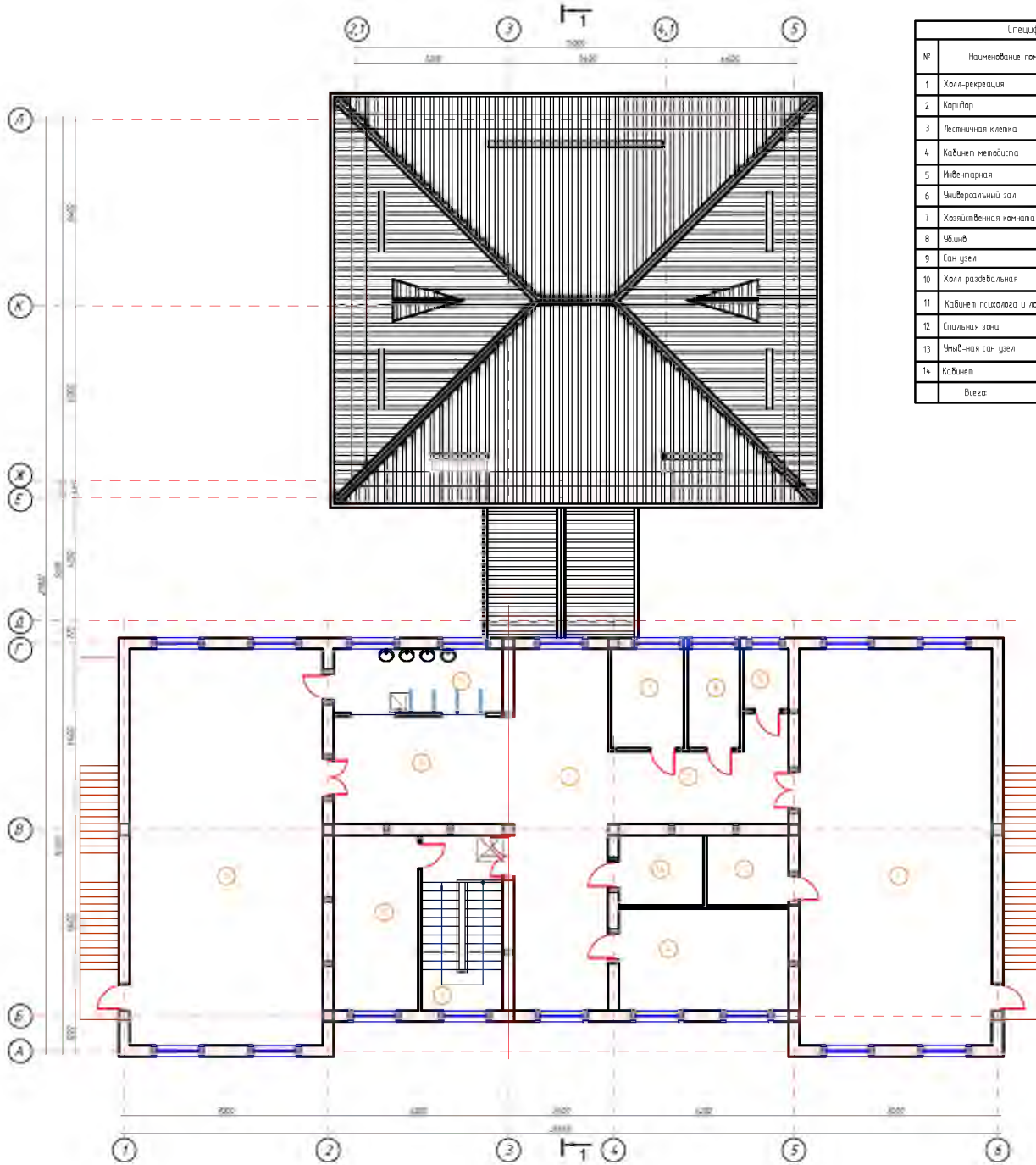
ПЛАН СТЕН 2го-ЭТАЖА М 1:100
