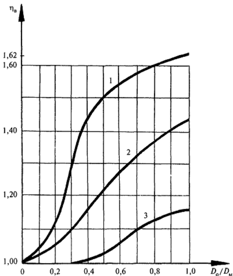
График для определения коэффициента несущей способности тройниковзв
