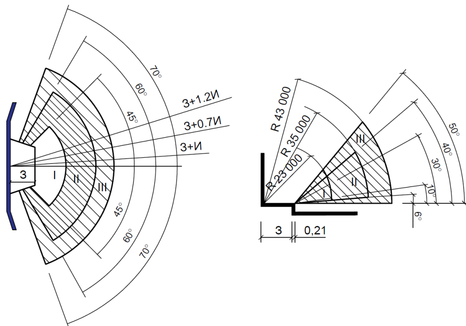
2-расм. Эстрада залида очилган сахна олдидаги томошабинлар жойлари
