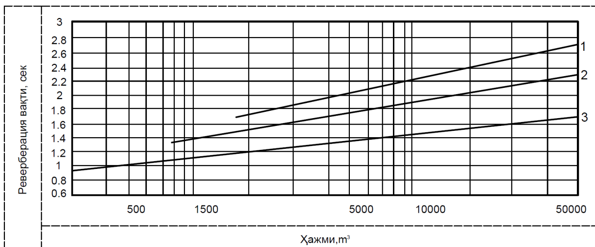
2-Расм 500 Гц дан 2000 Гц гача бўлган частоталарда ҳар хил мақсаддаги заллар учун уларнинг ҳажмига қараб тавсия этиладиган реверберация вақти
