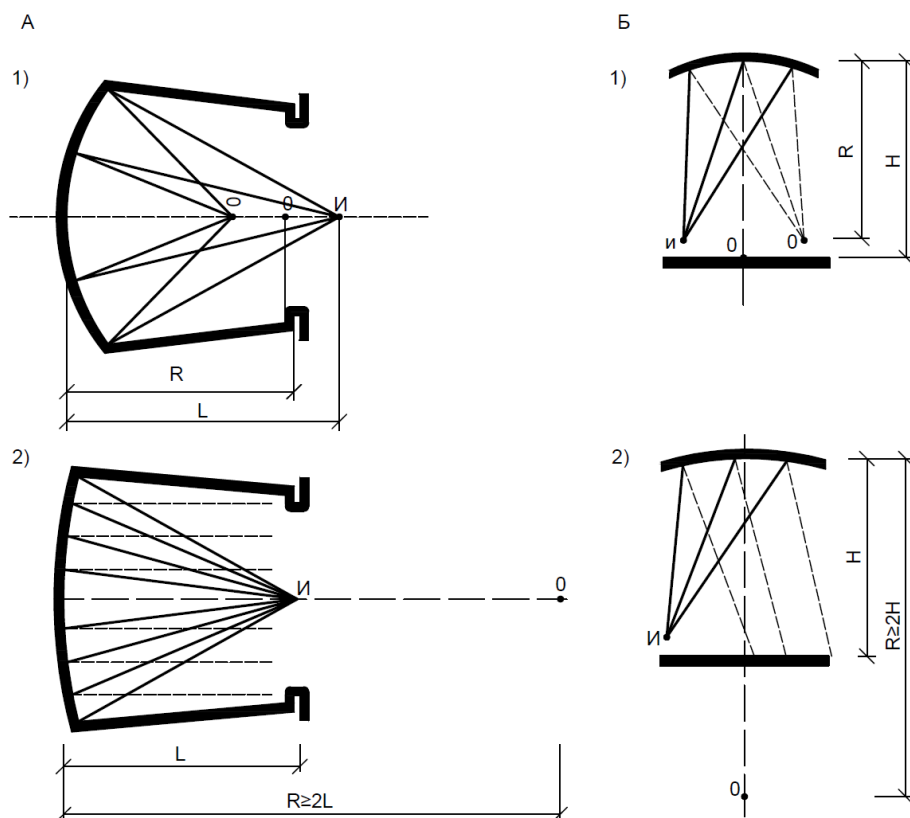
6-расм. Эгри юзалардан акс этиш
