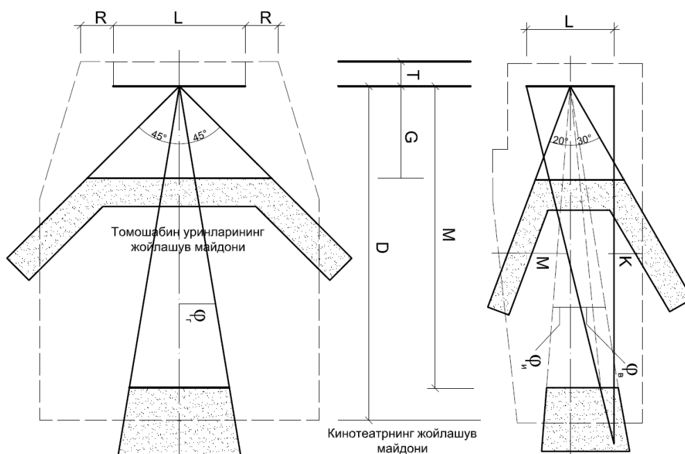
1-расм. Киноэкран ва томошабинлар залининг кўрсаткичлари
