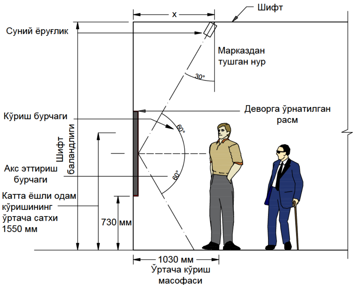
1-расм. Ёруғлик параметрлари
