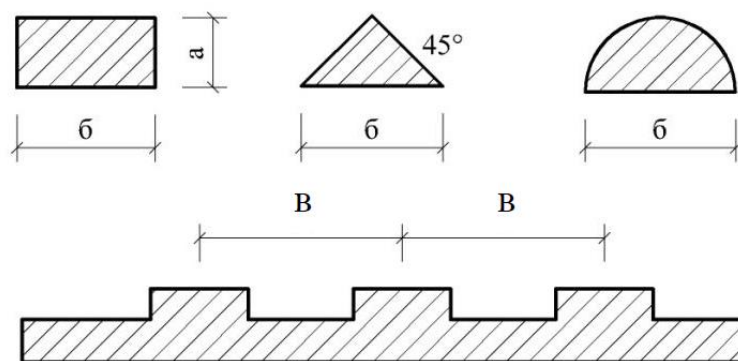
4-расм. Диффузли акс эттирувчи сиртнинг бўлиниш ўлчамлари
