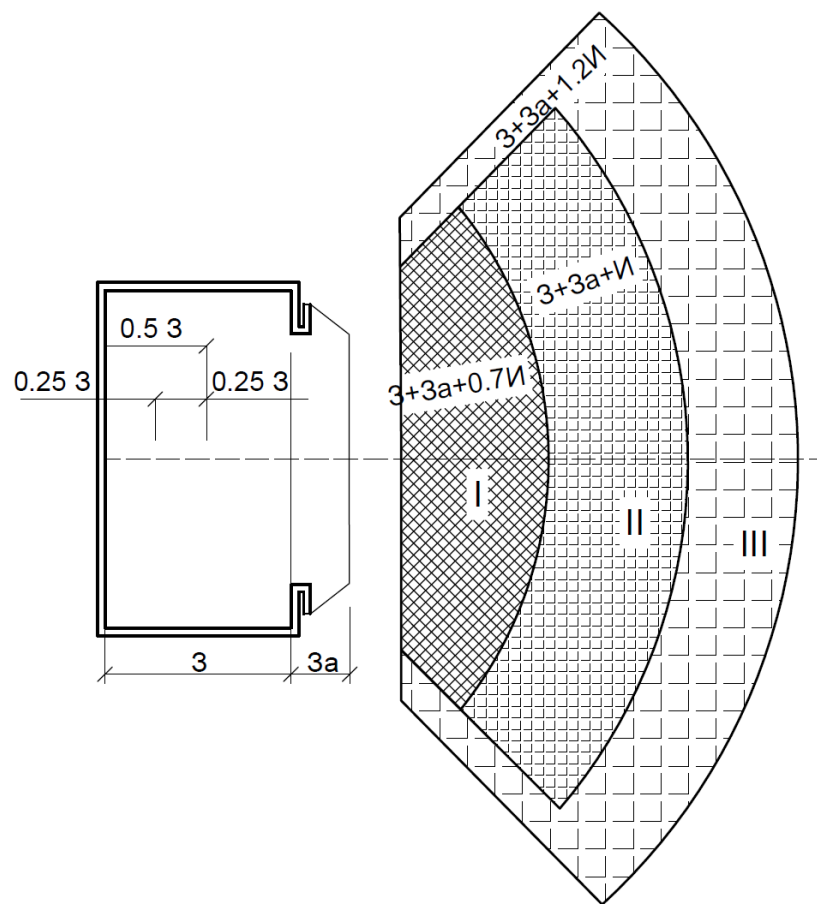
5-расм. Эстрада портали олдидаги томошабинлар жойлашуви зонаси режаси
