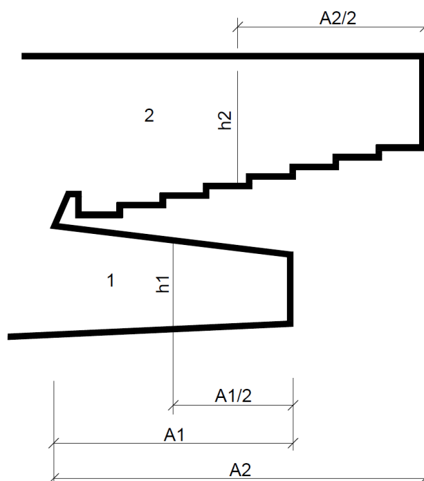
5-расм. Балкон бўшлигининг мақбул нисбатлари
