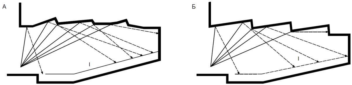
3-расм. Шифт юзасининг шакли
