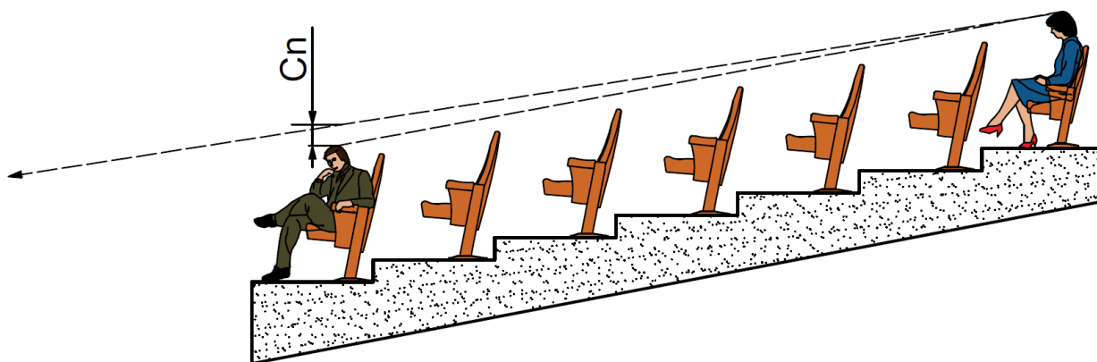
4-расм. Пол профилини кесиш учун кўриш нурининг C_p дан ошиши
