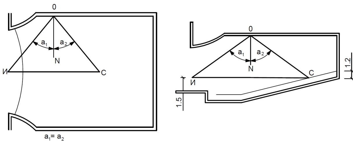
1-расм. Тўғридан-тўғри овоз схемаси.
