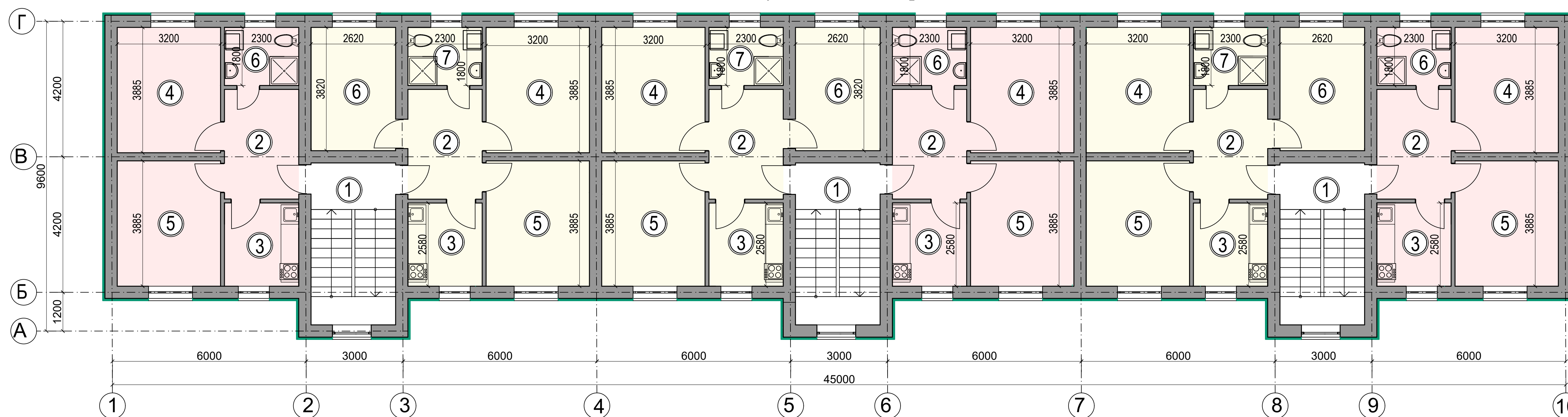
Намунавий қават тархи
