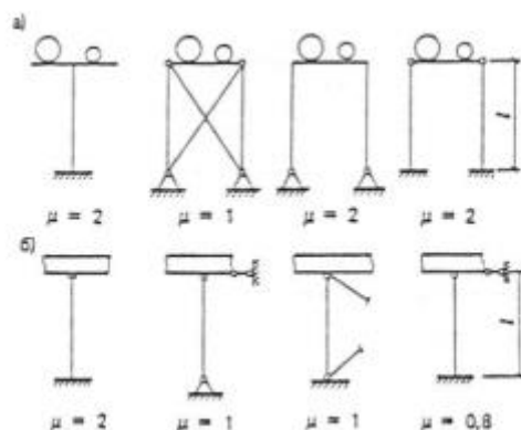
5-чизма. Кўп ярусли пўлат таянчларнинг ҳисобий схемалари а — оралик таянч; б — анкер таянч
